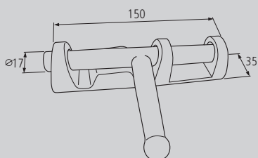
CERROJO FORJADO N°61 (PEQUEÑO) MANGO CORTO FORGED BOLT No. 61 (SMALL) SHORT HANDLE
